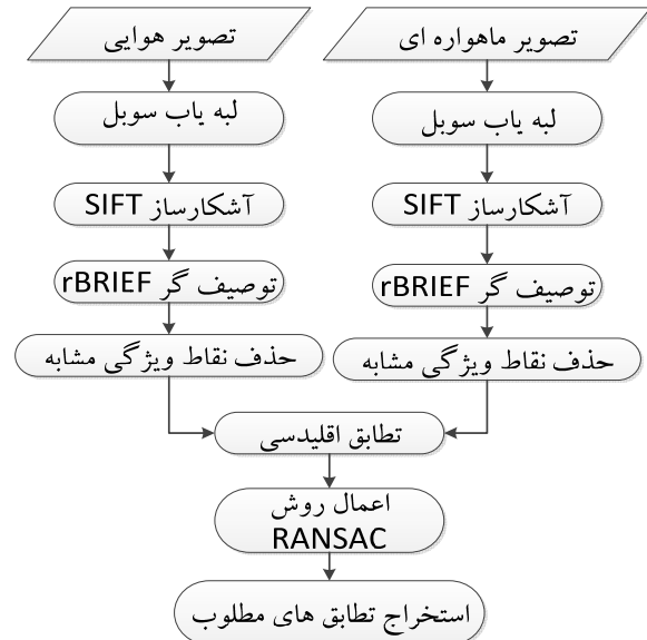
شکل ۱۰: روند نامی روش پیشنهادی در این تحقیق برای تطابق تصاویر هوایی و ماهواره‌ای.
