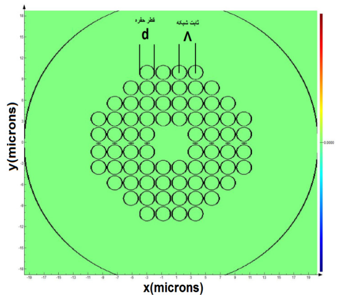
شکل ۱: نمایی از سطح مقطع فیبر بلور فوتونی پیشنهادی اولیه با قطر d = 2000 \text{ nm} و ثابت شبکه \Lambda = 2200 \text{ nm} .
