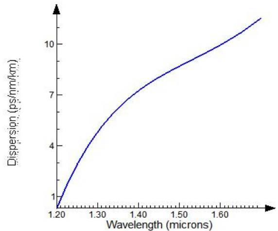
شکل ۶: نمودار پاشندگی بر حسب طول موج در فیبر بلور فوتونی پیشنهادی تکمیلی.
