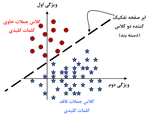
شکل ۱: واژه‌یاب گفتار به عنوان یک دسته‌بند دودویی.
