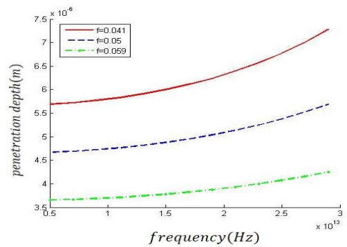
شکل ۸: طول انتشار (الف) و عمق نفوذ (ب) بر حسب فرکانس با تغییر مقدار پراشگی برای دی الکتریک پوشش از جنس دی اکسید سیلیکون.
