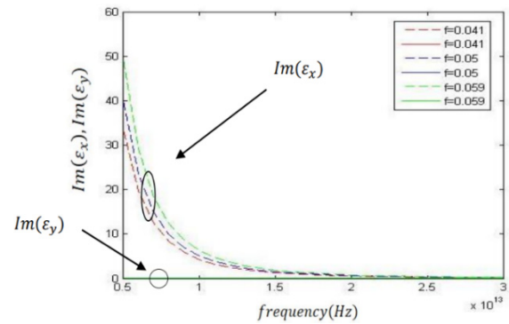
شکل ۶: قسمت موهومی ضریب گذردهی پوشش بر حسب فرکانس برای مقادیر مختلف پراشگی.
