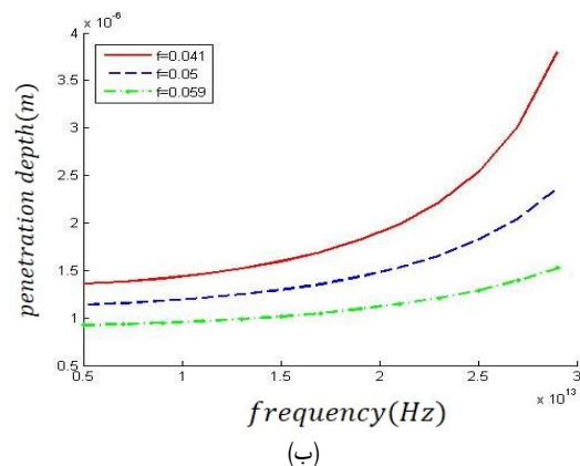
شکل ۷: طول انتشار (الف) و عمق نفوذ (ب) بر حسب فرکانس با تغییر مقدار پراشگی برای دی الکتریک پوشش از جنس سیلیکون.
