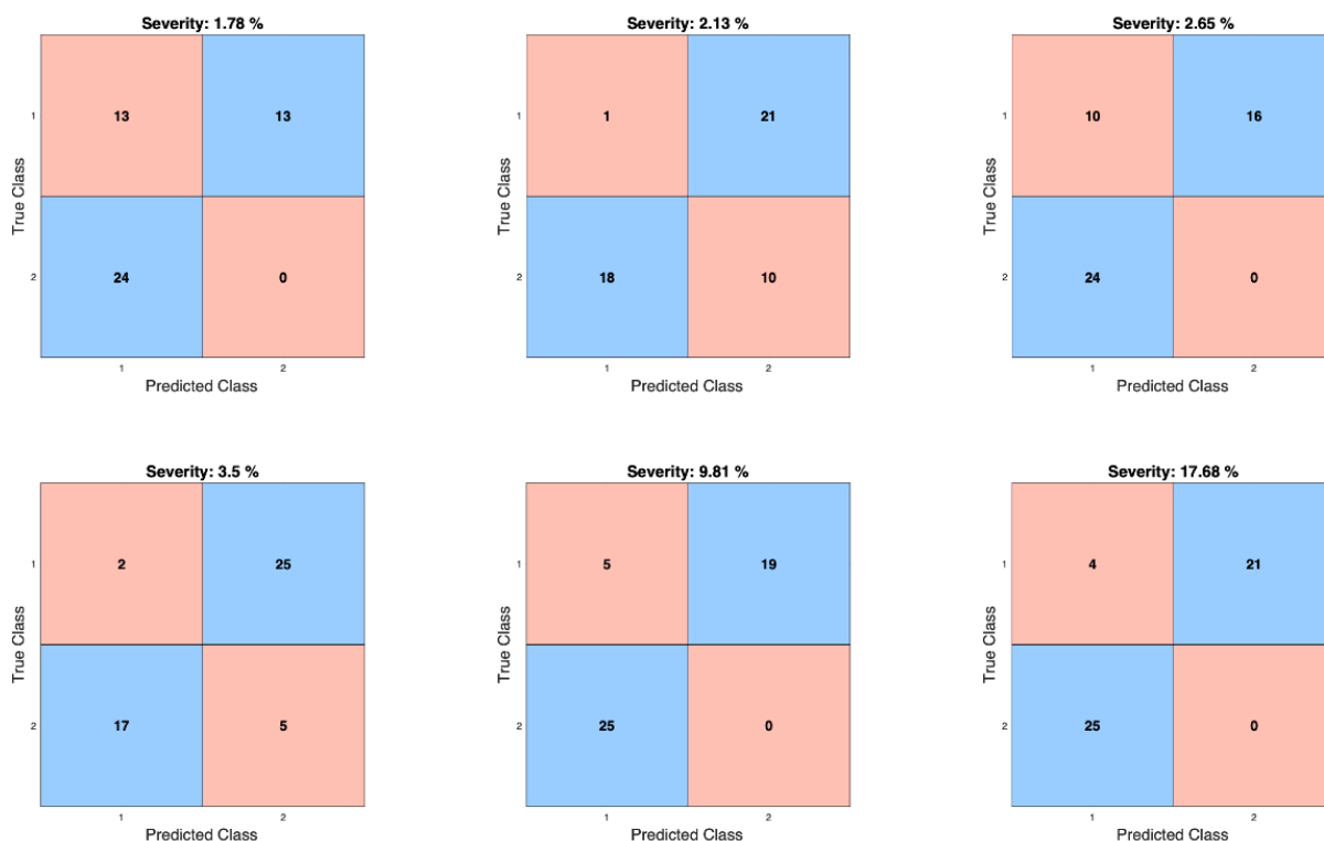
شکل ۱۶: ماتریس‌های سردرگمی الگوریتم LSTM [۴۴] در مرحله آزمون برای طبقه‌بندی شدت عیوب مختلف.
