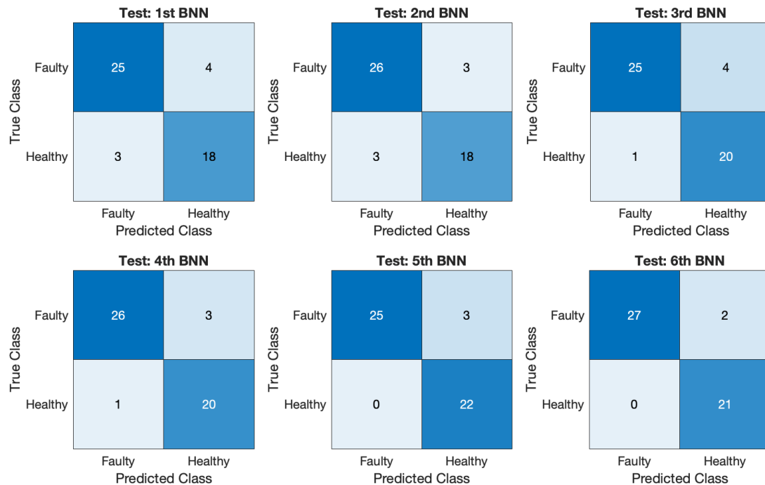
شکل ۱۴: ماتریس‌های سردرگمی برای مدل‌های BNN در مرحله آزمون مربوط به شدت‌های ۱/۷۸٪، ۲/۱۳٪، ۳/۶۵٪، ۳/۸۱٪ و ۱۷/۶۸٪.
