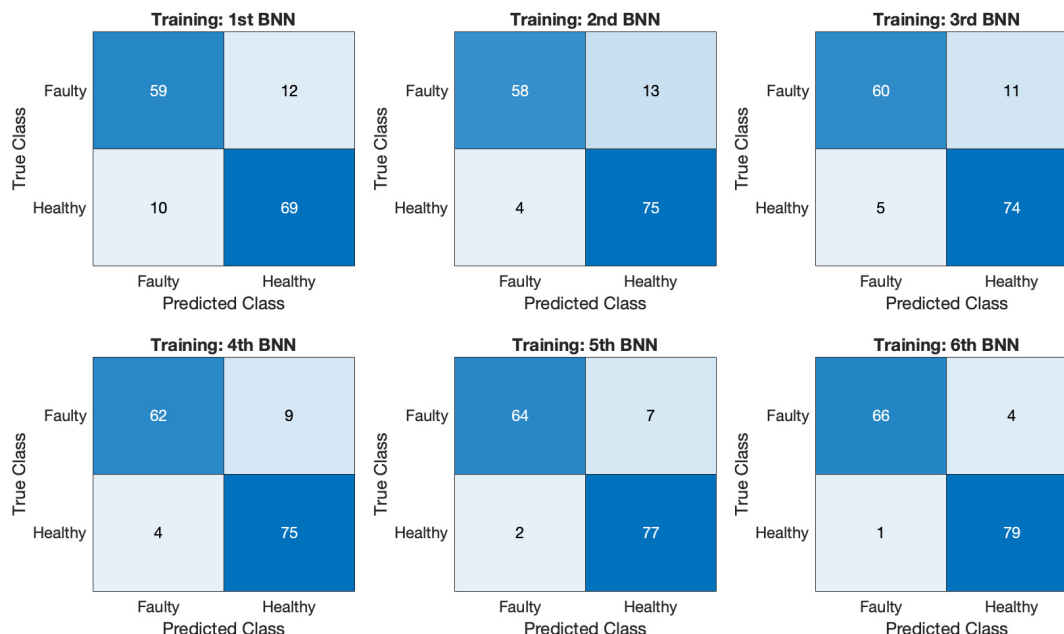
شکل ۱۳: ماتریس‌های سردرگمی برای مدل‌های BNN در مرحله آموزش مربوط به شدت‌های ۱، ۲، ۳، ۴، ۵ و ۶، ۷، ۸، ۹، ۱۰ و ۱۱، ۱۲، ۱۳، ۱۴، ۱۵ و ۱۶٪.
