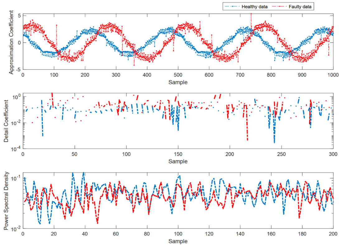
شکل ۳: PSD و DWT سیگنال‌های جریان سه فاز برای داده‌های سالم و معیوب با شدت عیب ۹/۸۱٪.
