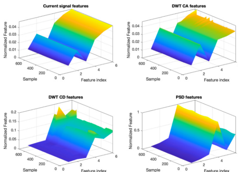
شکل ۴: توزیع ویژگی‌ها برای داده‌های سالم و معیوب با شدت عیب مختلف.
